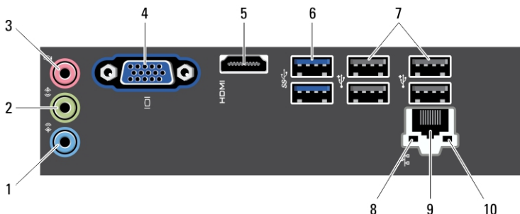
Slika 2. Zadnja ploča
